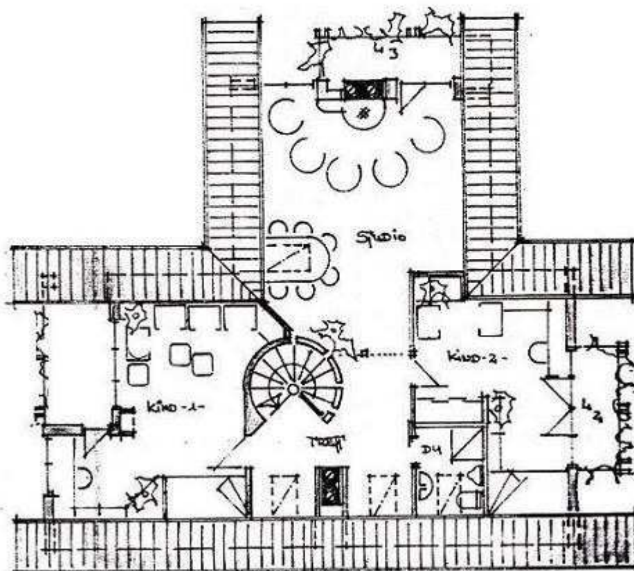
Dachgeschoss
